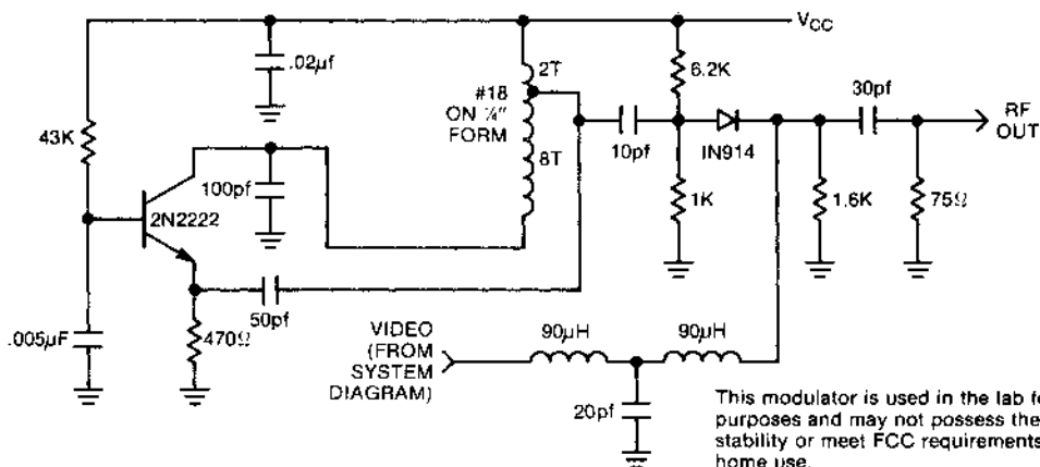
Fig.8 VHF MODULATOR
