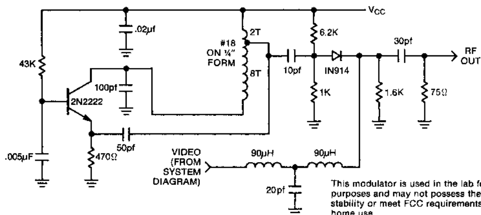
Fig.8 VHF MODULATOR
