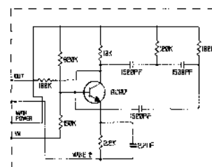
Fig. 20 SINE-WAVE OSC
