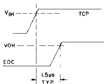
Fig.39 EOC TURN-ON
