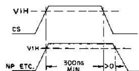
Fig.15b CS
