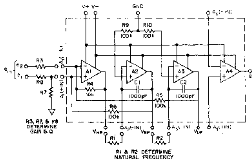
Fig. 1 SCHEMATIC
