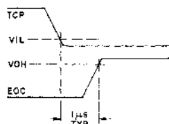
Fig.17 EOC TURN-ON
