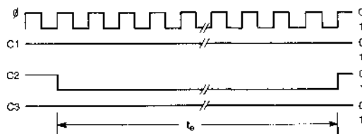
Fig.4 ERASE
